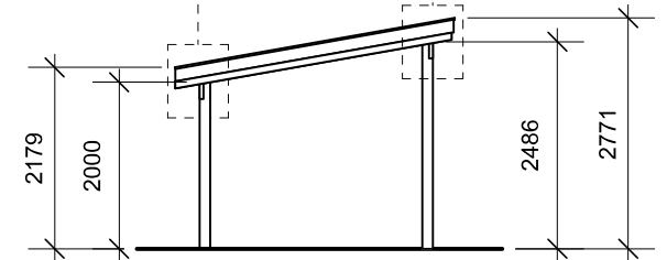
Gavl
