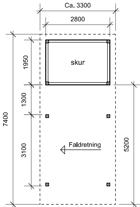
Plantegning
