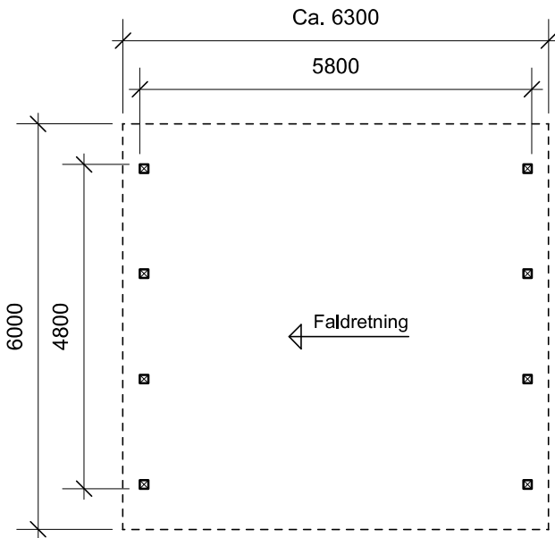
Plantegning
