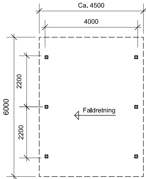
Plantegning
