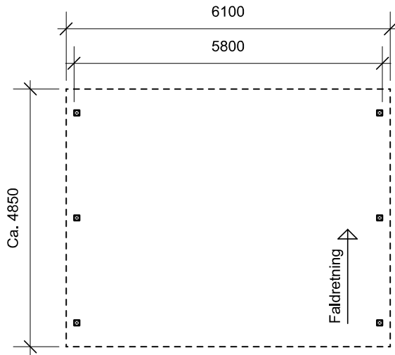
Plantegning
