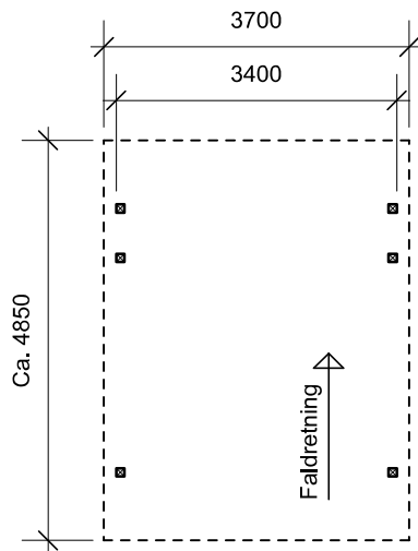
Plantegning
