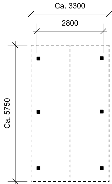
Plantegning
